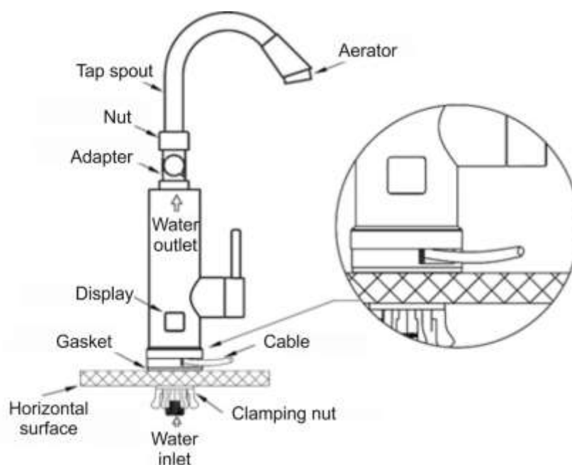
1. slika. Izlaz kabla za napajanje iznad sudopere
