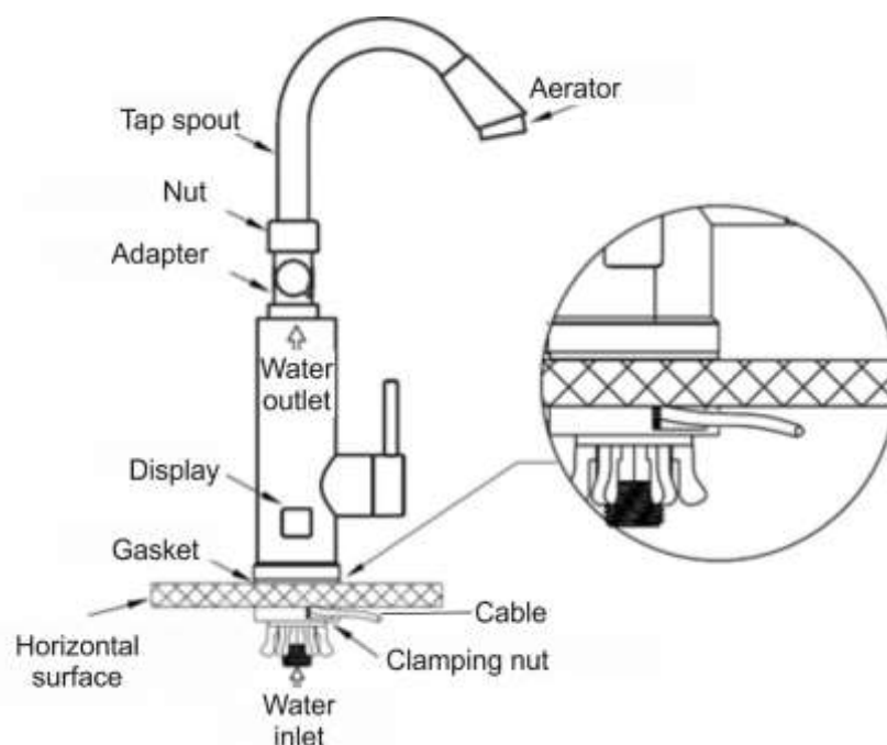
2. slika. Izlaz kabla za napajanje ispod sudopere
